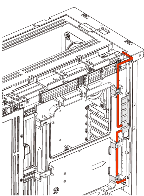
5 Fan cable channel
