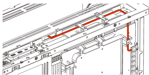
3 Fan cable channel
